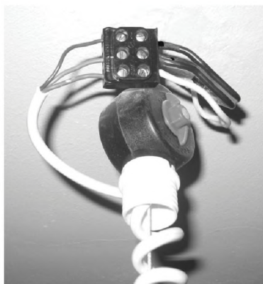
Рис. 94. Альтернативные варианты соединения электрических проводов от квартирной проводки к люстре
