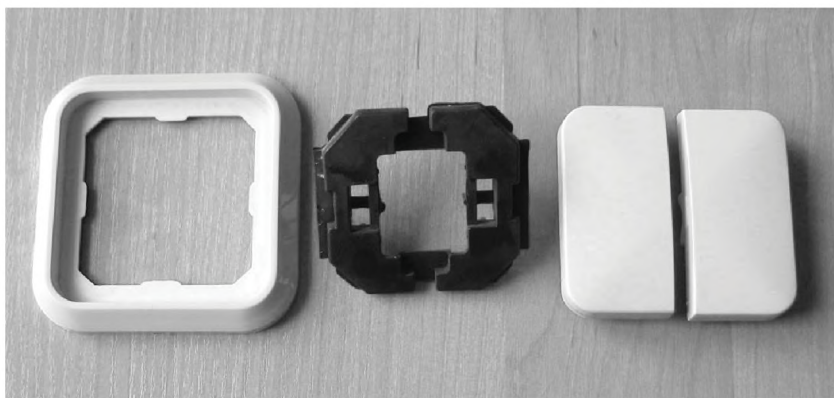
Рис. 59. Части двухклавишного выключателя
