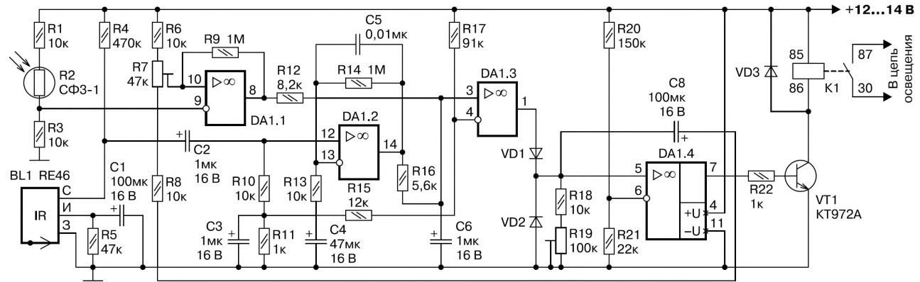
Рис. 37. Электрическая схема промышленного датчика движения
