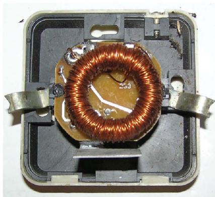
Рис. 97. Вид на диммер и элементы крепления – со снятой крышкой корпуса
