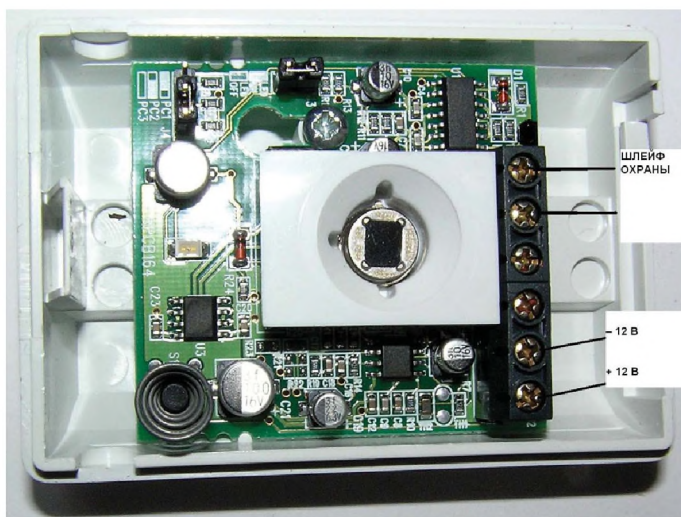
Рис. 47. Вид со снятой крышкой корпуса датчика «Фотон-9»
